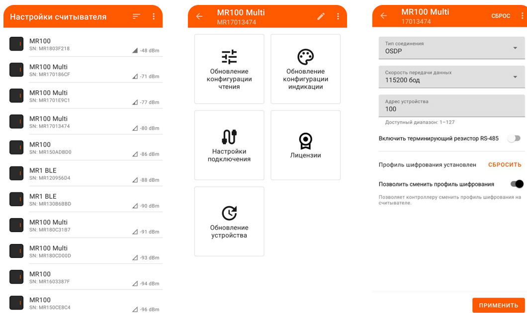
Процесс активации опции «Позволить сменить профиль шифрования».
